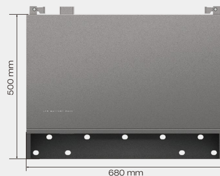
Batteria LFP EcoFlow PowerOcean (installazione a parete)
