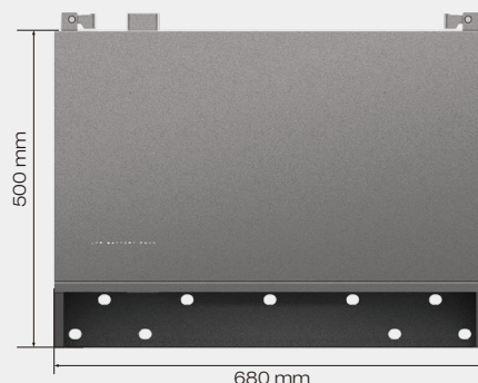
Bateria LFP EcoFlow PowerOcean (ze wspornikiem do montażu na ścianie)
