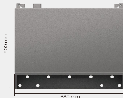
Batería LFP EcoFlow PowerOcean (con montaje en pared)
